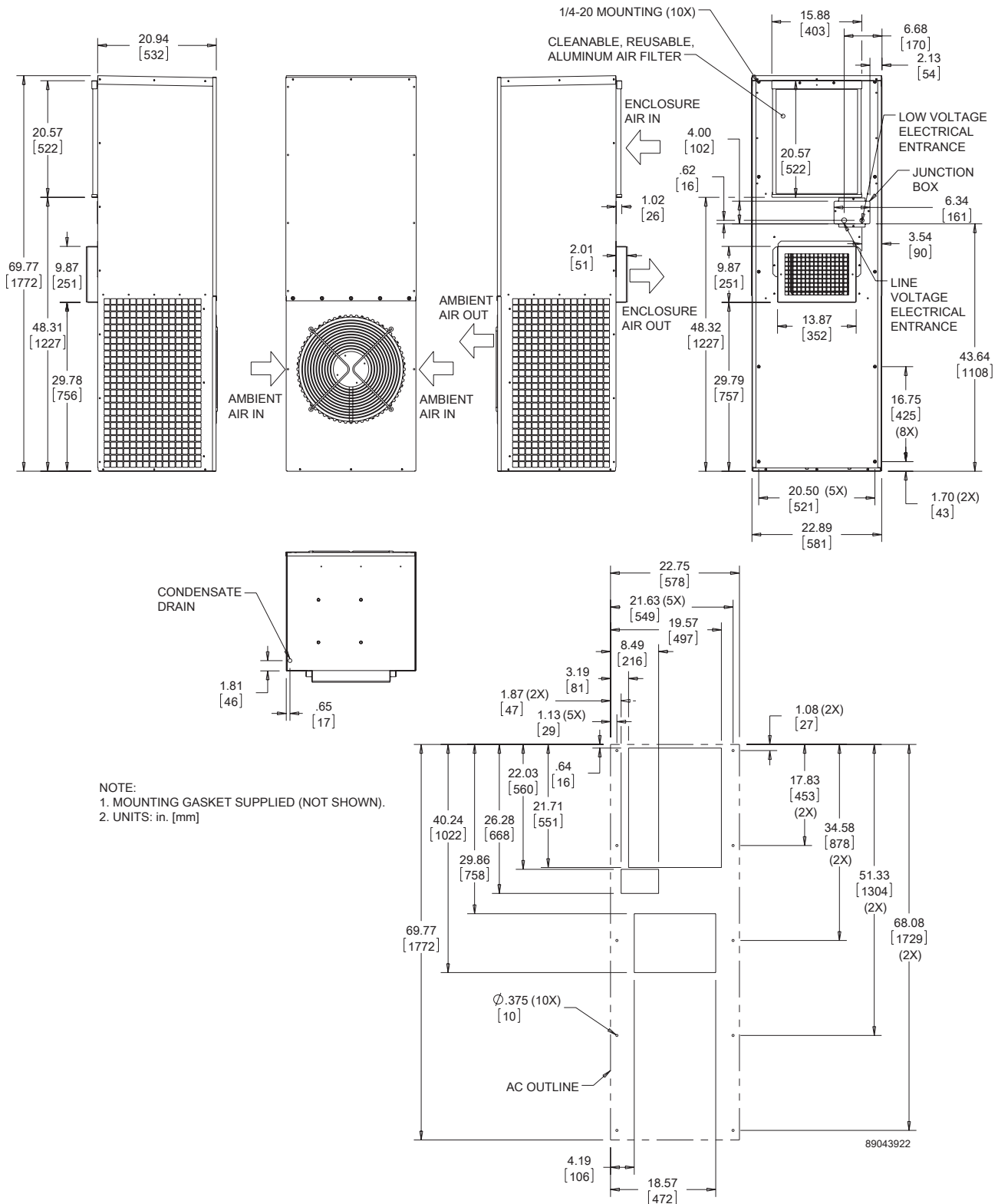
Cutout Dimensions
